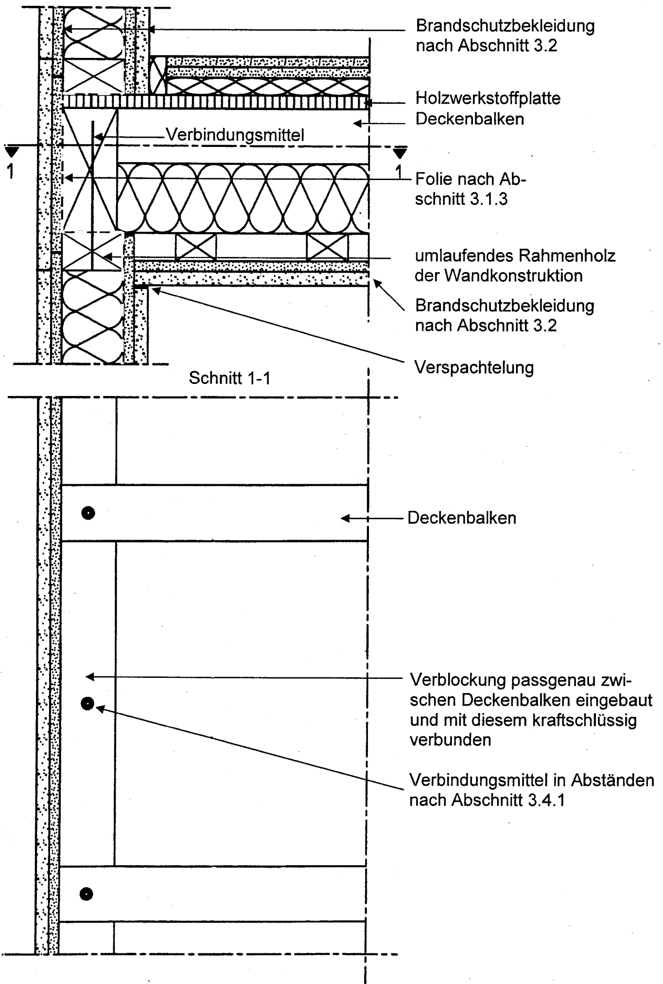
Bild 1 Anschluss Decke nach Abschn. 3.3.3 an tragende und raumabschließende Wand nach Abschn. 3.3.2 mit Brandschutzbekleidung nach Abschn. 3.2 (z. B. Trepperraumwand, Außenwand – Spannrichtung der Deckenbalken senkrecht zur Wand)
